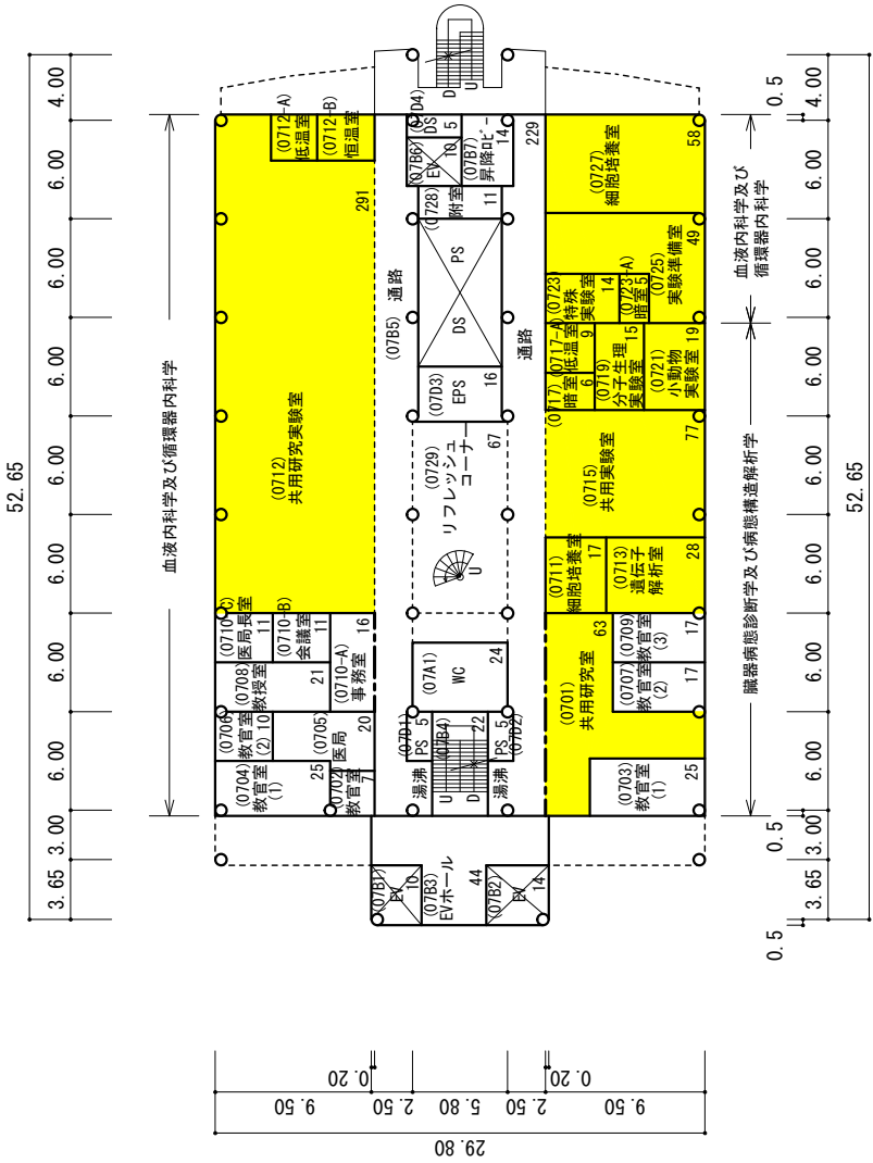
7 階 1,307㎡ S=1/500
